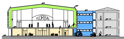
řez halou a atriem
