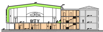
řez halou v místě vstupu a spojovacího krčku
